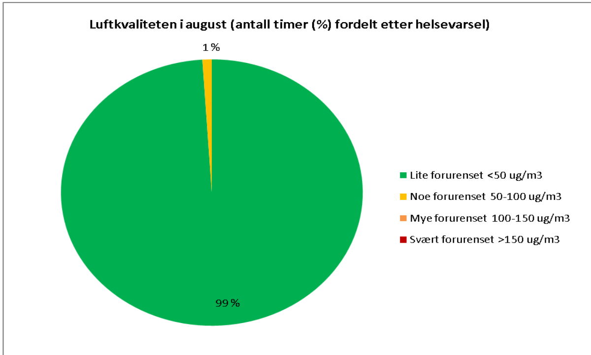
Figur 2. Figuren viser hvor mange prosent av tiden hvor luftkvaliteten i august har ligget innenfor de ulike helsevarsel.
