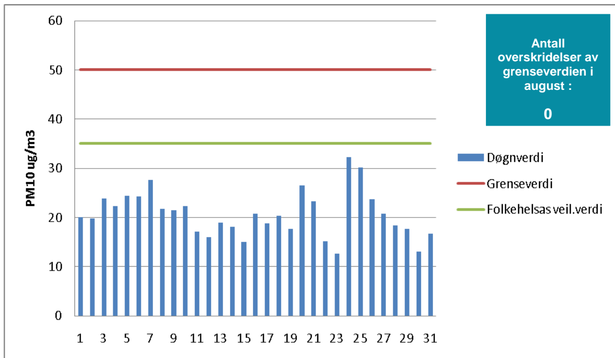
Figur 1. Døgnmiddel av svevestøv \text{PM}_{10} (partikkelstørrelse) målt i St.Croix-krysset i august 2009. Grunnet ferieavvikling er det ikke registrert nedbørsdata for denne perioden.
