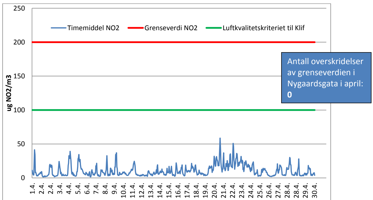
Figur 3 Timemiddelkonsentrasjon av nitrogendioksid ( NO_2 ) målt i Nygaardsgt i april 2015. Stasjonen har vært i normal drift i hele perioden.
