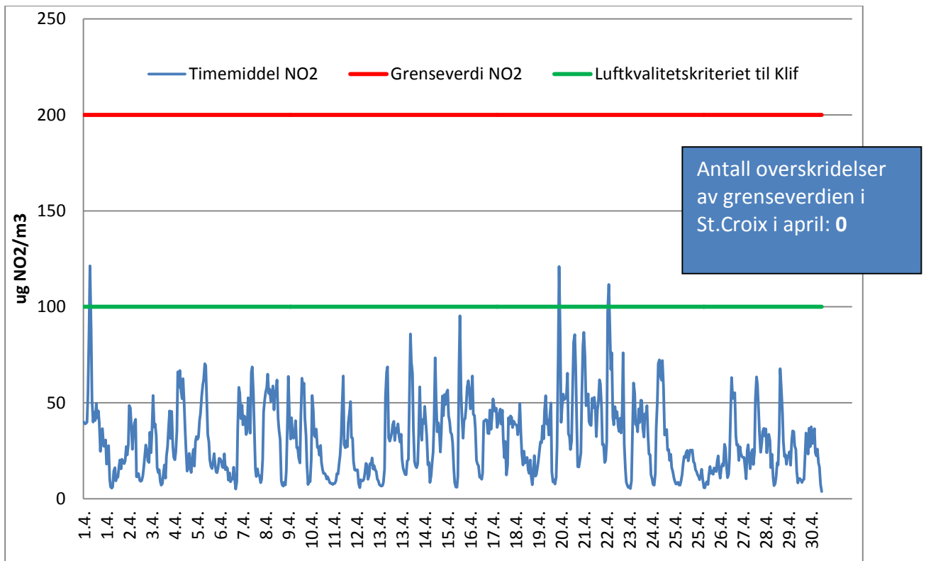
Figur 4. Timemiddelkonsentrasjon av nitrogendioksid (NO 2 ) målt i St.Croix i april 2015. Stasjonen har vært i normal drift i hele perioden.
