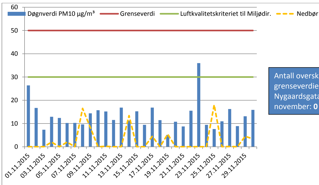
Figur 1 Døgnmiddelkonsentrasjon av svevestøv (PM 10 ) målt i Nygaardsgt i november 2015. Stasjonen har vært i normal drift i hele perioden.
