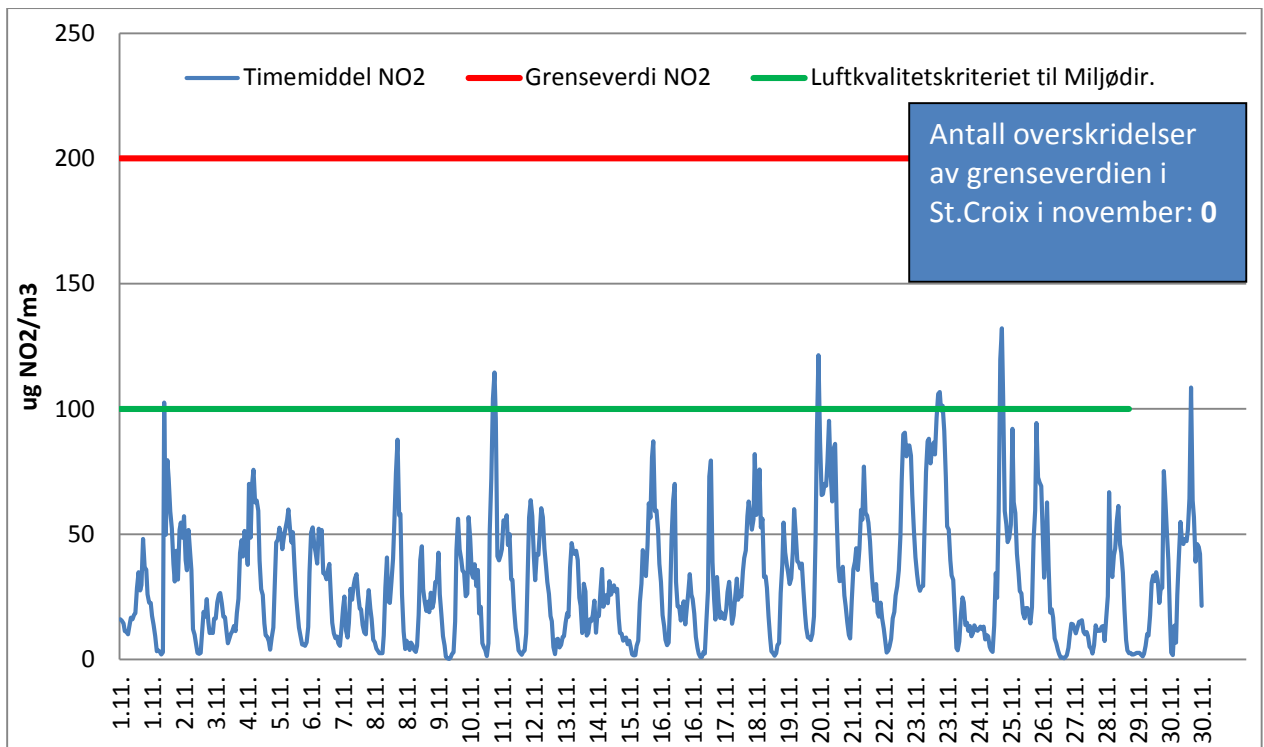
Figur 4. Timemiddelkonsentrasjon av nitrogendioksid (NO 2 ) målt i St.Croix i november 2015. Stasjonen har vært i normal drift i hele perioden.
