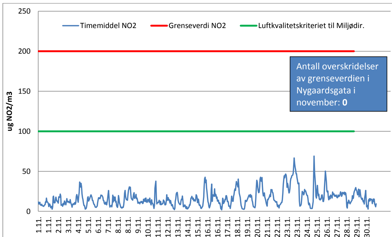
Figur 3 Timemiddelkonsentrasjon av nitrogendioksid ( NO_2 ) målt i Nygaardsgt i november 2015. Stasjonen har vært i normal drift i hele perioden.
