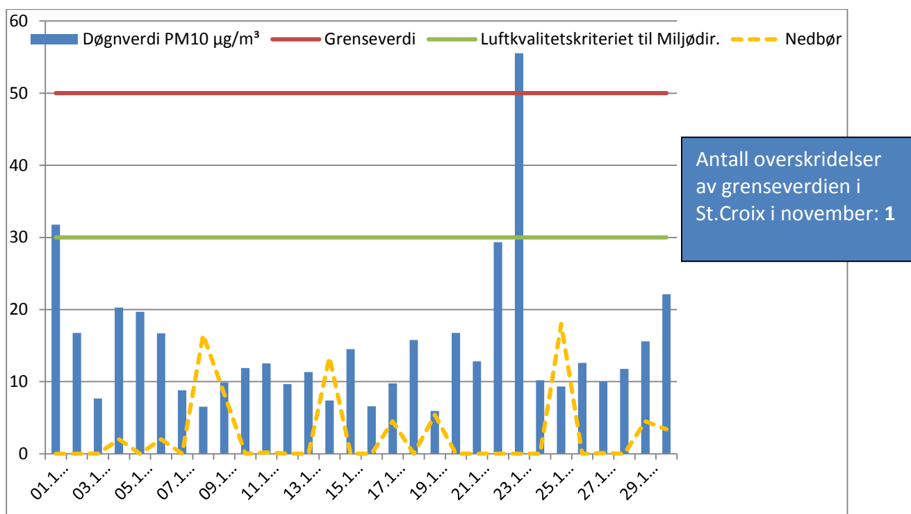
Figur 2 Døgnmiddelkonsentrasjon av svevestøv ( PM_{10} ) målt i St.Croix i november 2015. Stasjonen har vært i normal drift i hele perioden.
