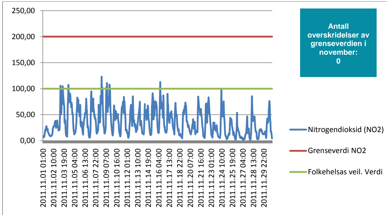
Figur 2. Timemiddelkonsentrasjonen av nitrogendioksid (NO 2 ) målt i St.Croix-krysset i november 2011. Stasjonen har vært i normal drift i hele perioden.
