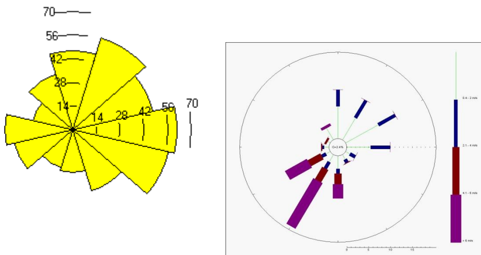
Figur 4. Som det fremgår av figuren til høyre var dominerende vindretning i november fra sørvest og nordøst (meteorologidata fra Borge). Høyeste vindhastighet forekommer ved vind fra sørvest. Figuren til venstre viser forholdet mellom vindretning og svevestøvkonsentrasjon. Høyeste konsentrasjoner forekommer ved vindretning fra nordøst og øst når vindhastigheten er lav.
