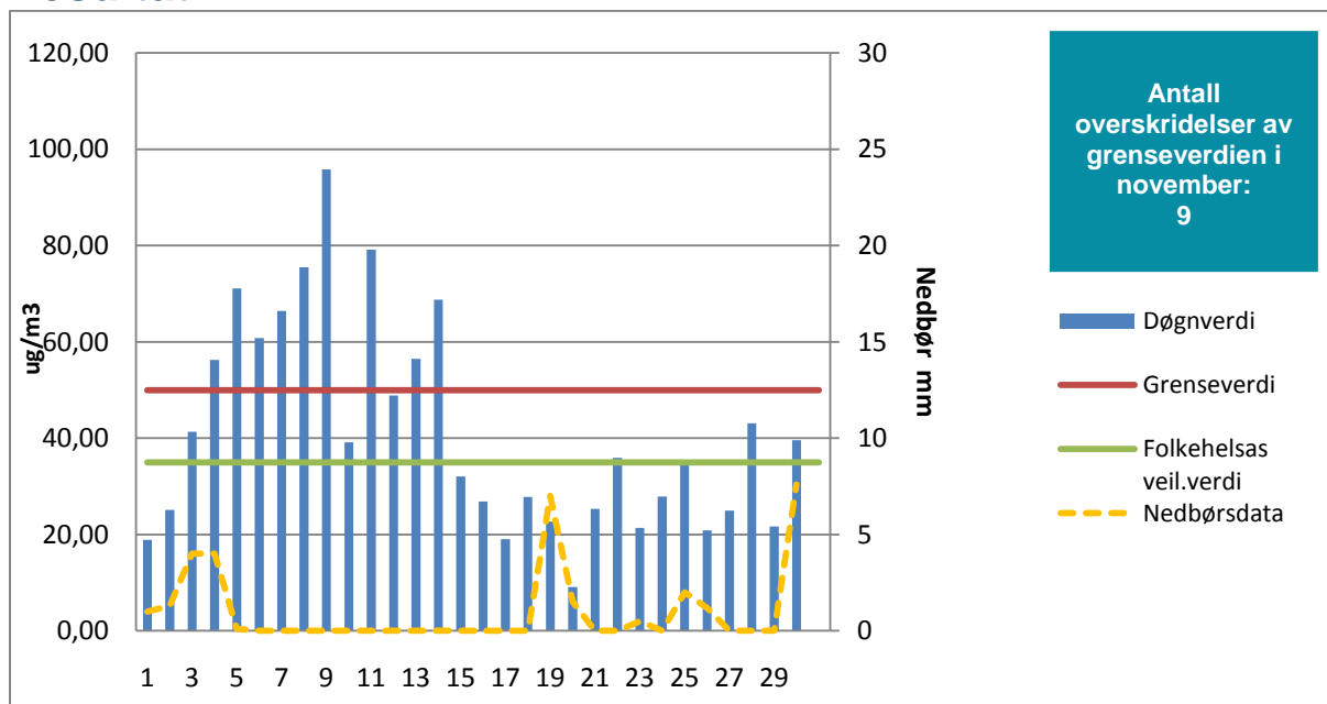
Figur 1. Døgnmiddel av svevestøv PM 10 (partikkelstørrelse) målt i St.Croix-krysset i november 2011. Stasjonen har vært i normal drift i hele perioden
